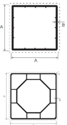
Pfosten hohl
