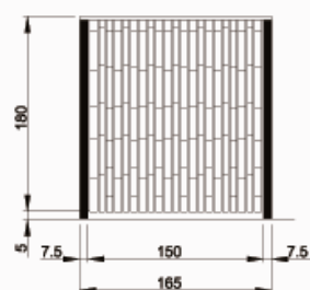
élément complet l. 150 cm
