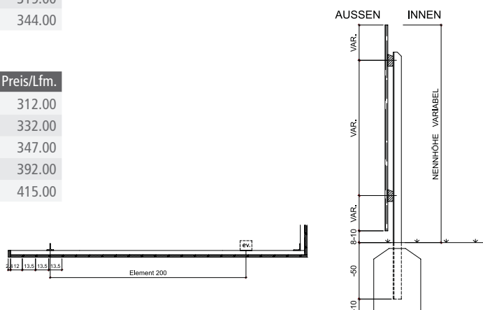
Ansicht aussen
